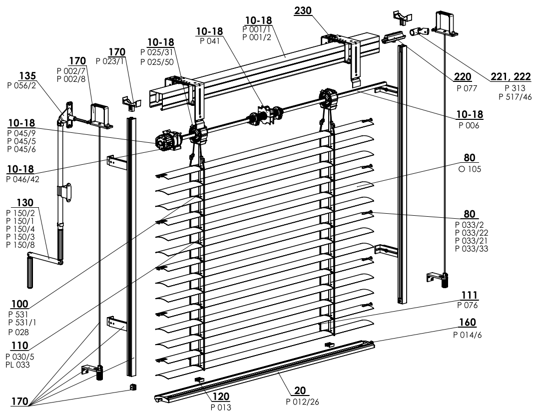
FLEXI 60 - KLIKA
