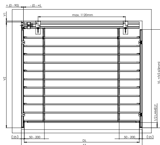
vedení vodící lištou - kolmá
