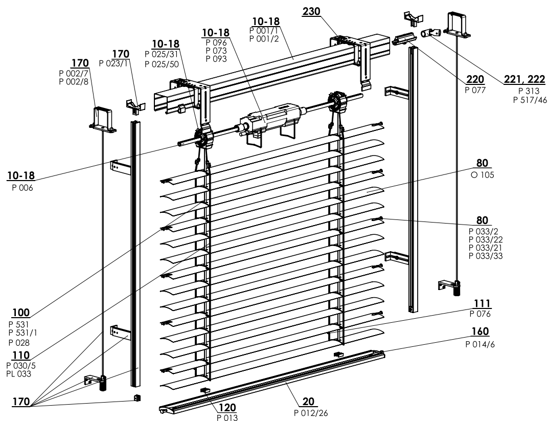
FLEXI 60 - MOTOR
